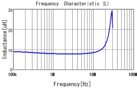
■ 1267AY-100M L
