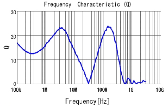
■ 1267AY-100M Q
